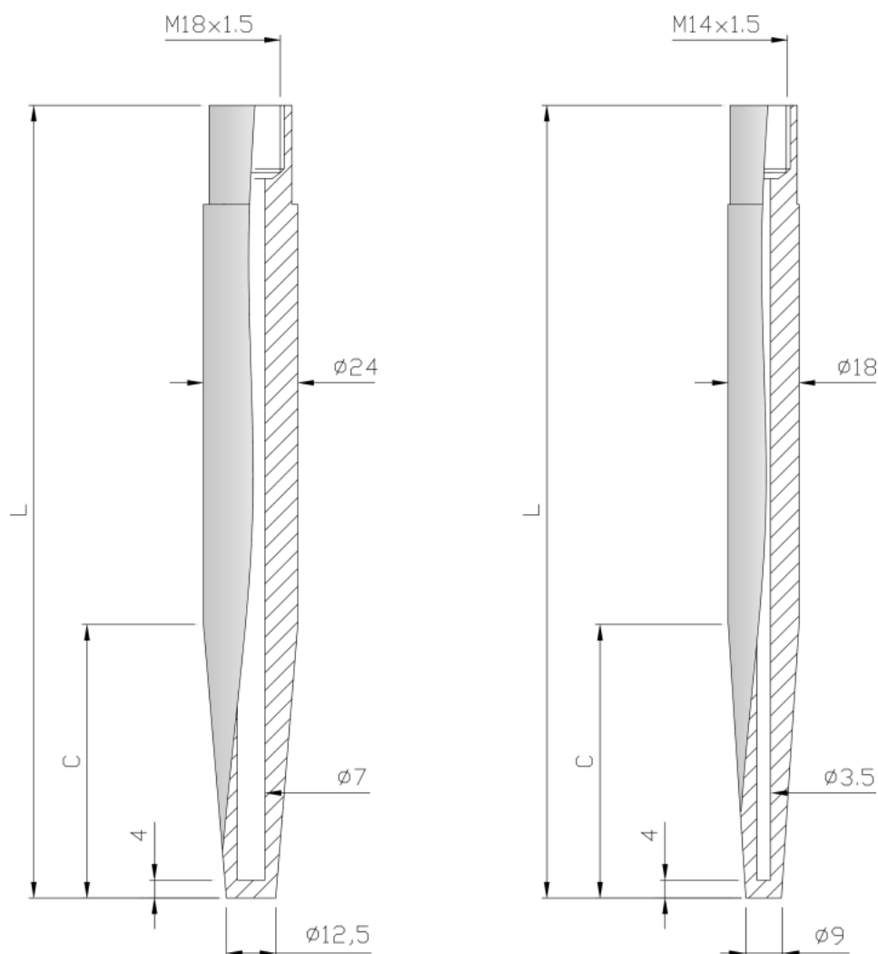
Oślona ciśnieniowa typu D DIN 43 763
